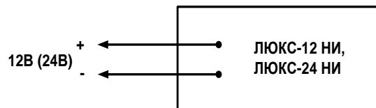
Рис.1. Схема подключения.
